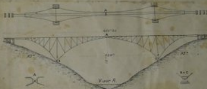
VUE SCHEMATIQUE DU VIADUC, EN PLAN ET EN ELEVATION
