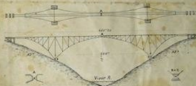
VUE SCHEMATIQUE DU VIADUC, EN PLAN ET EN ELEVATION
